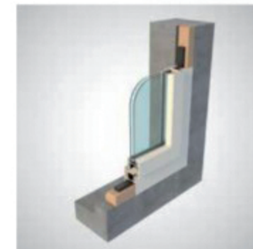
Pose en rénovation
