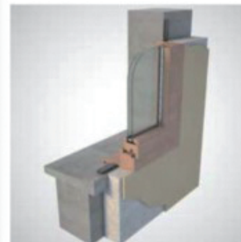
Pose en applique
