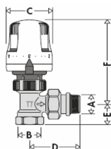
Equerre
