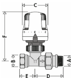
Droit
